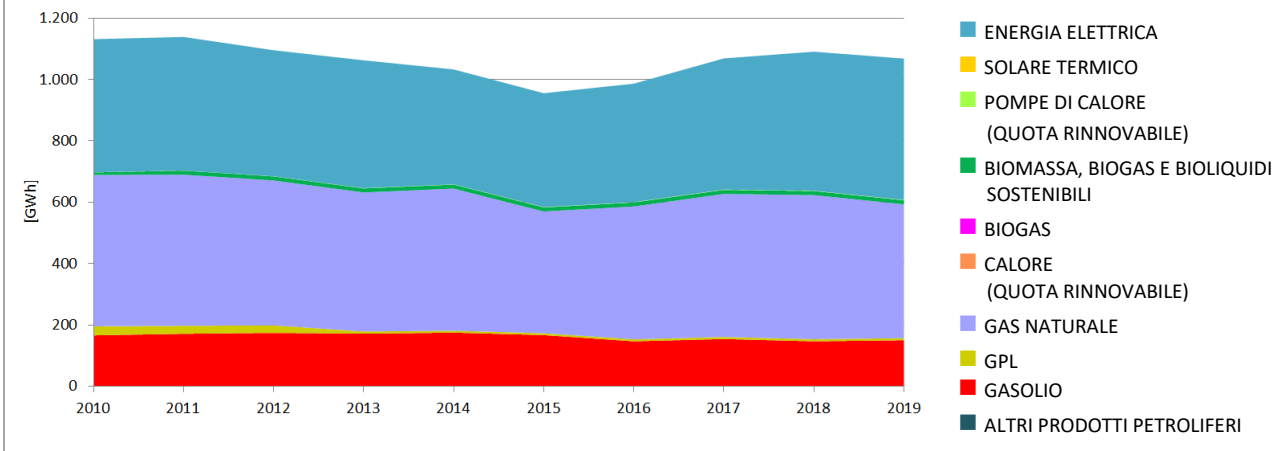
GRAFICO 65 – ANDAMENTO CONSUMI FINALI NETTI - SETTORE INDUSTRIA/AGRICOLTURA - PER VETTORI (2010-2019) [Fonte: BER]
