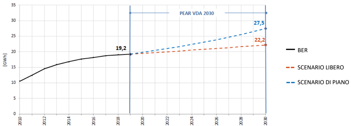
GRAFICO 118 – SOLARE TERMICO – PRODUZIONE - CONFRONTO TRA SCENARIO LIBERO E SCENARIO DI PIANO
