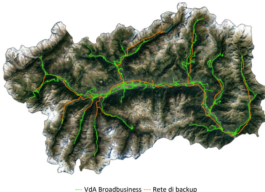
FIGURA 17 - Reti di fibra ottica (progetto Broadbusiness e rete di backup) [Fonte: Geoportale VdA]
