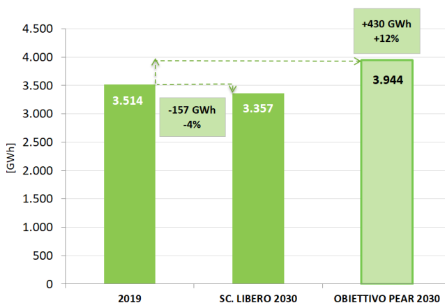
GRAFICO 89 – SCENARIO LIBERO – OBIETTIVO 2 – AUMENTO DALLE PRODUZIONE DA FER LOCALI
