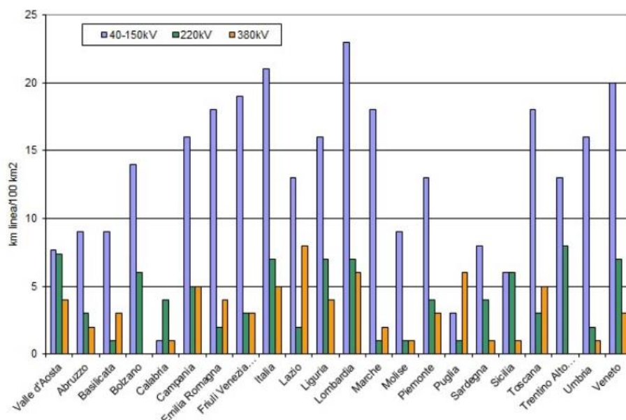
GRAFICO 38 – LUNGHEZZA DELLE LINEE ELETTRICHE AT e AAT NORMALIZZATA ALLA SUPERFICIE REGIONALE (km di linea/100km 2 ) - [Fonte: ARPA VdA - ISPRA]
