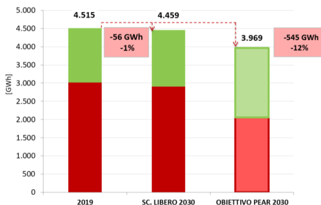
GRAFICO 88 – SCENARIO LIBERO – OBIETTIVO 1 –RIDUZIONE DEI CFN
