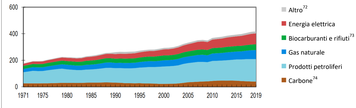
GRAFICO 19 – ANDAMENTO CONSUMI FINALI [EJ] MONDIALI PER FONTE (1971-2019)
