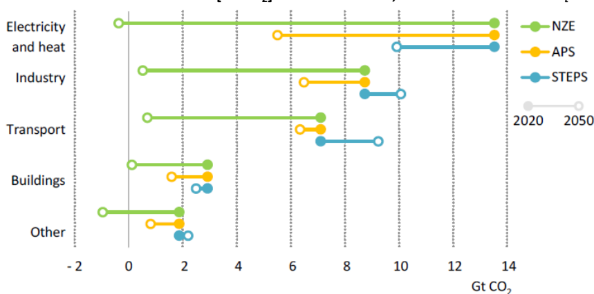
GRAFICO 22 – EMISSIONI - LIVELLO MONDIALE [Gt CO 2 ] – SCENARI STEPS, APS E NZE PER SETTORI [Fonte: IEA 2021c ]
