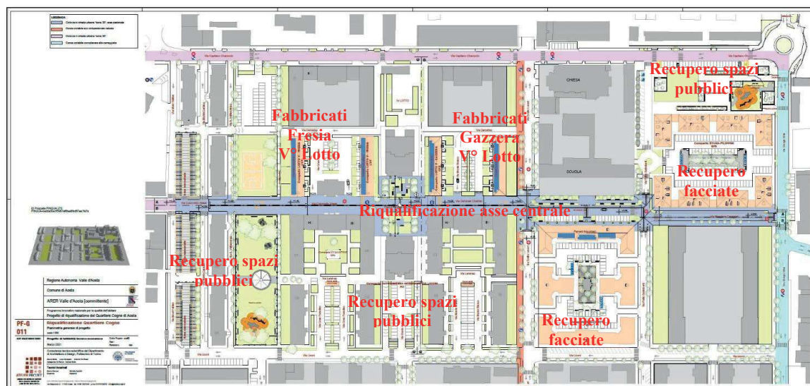
Figura 2 – Planimetria generale del Progetto
