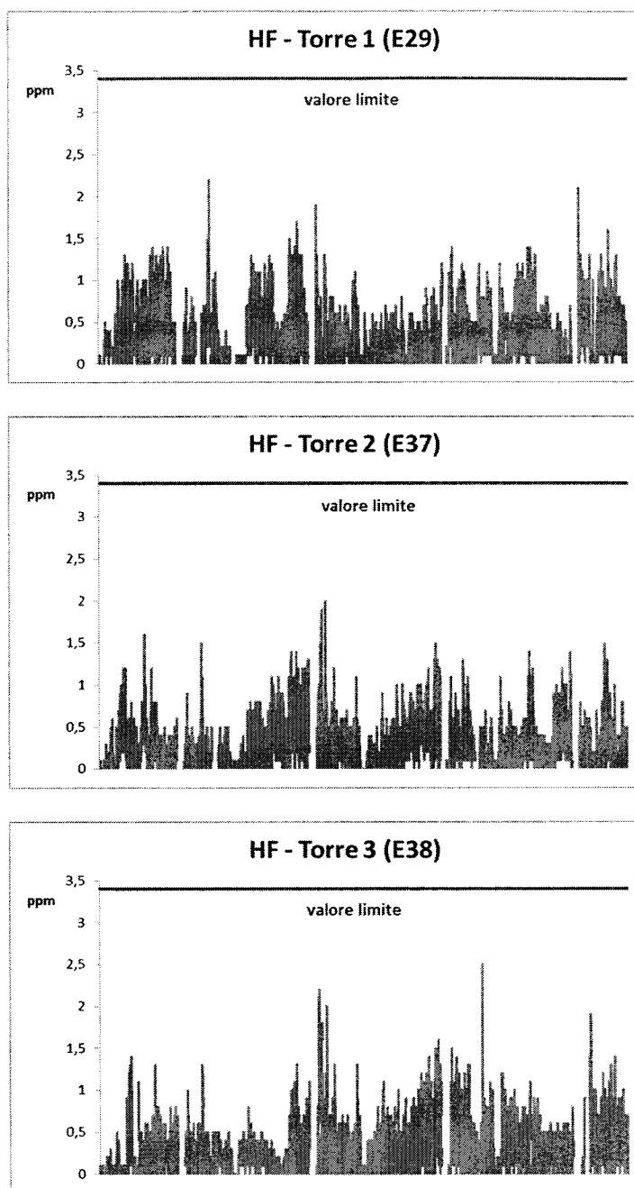
Figura 1 – Valori medi orari di emissione di HF rilevati dal misuratore automatico installato sulle prime 3 torri di lavaggio (periodo dal 01/01/2013 al 31/12/2015)
